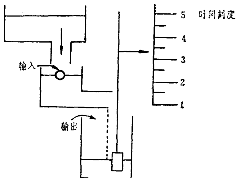
图1·1 水 钟
