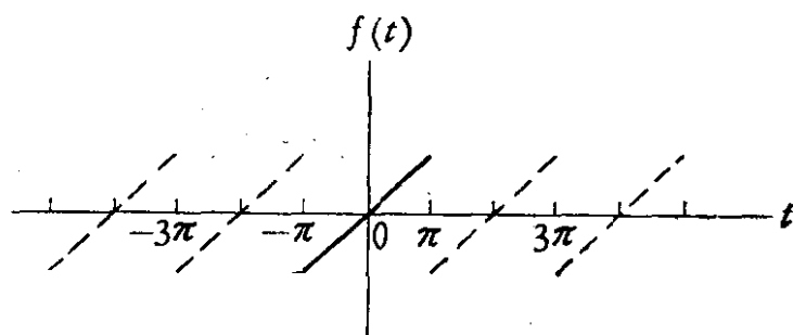
图 1.4 f(t)=t ( -\pi < t < \pi )
