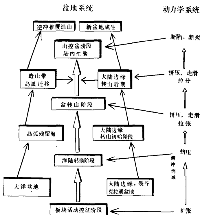
图 0-2 盆山转换过程分析
