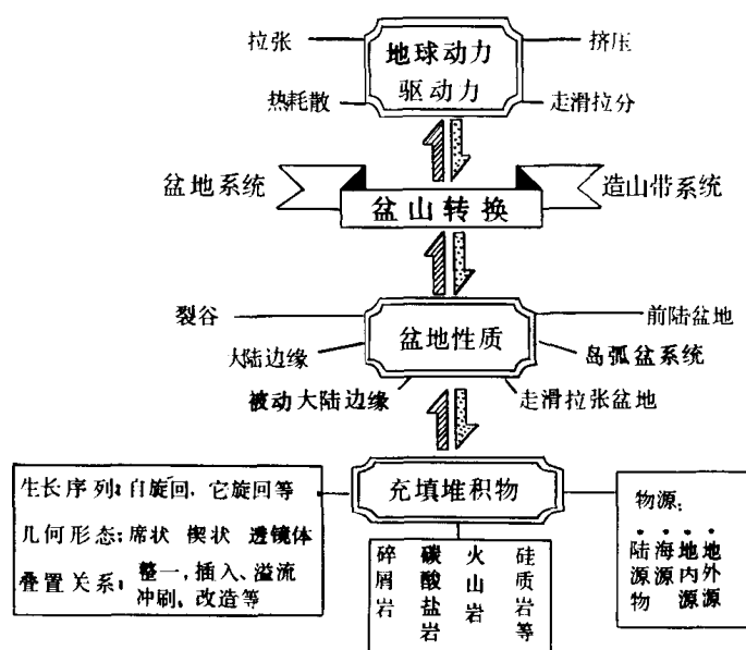
图 0-1 地球动力作用在盆地中的响应
