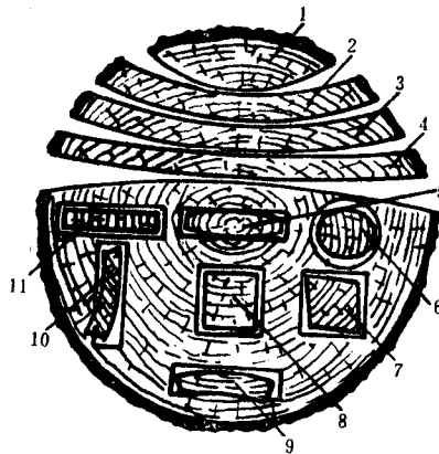
图 1-5 木材变形
