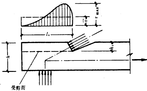
图 1-8 单齿剪切应力
