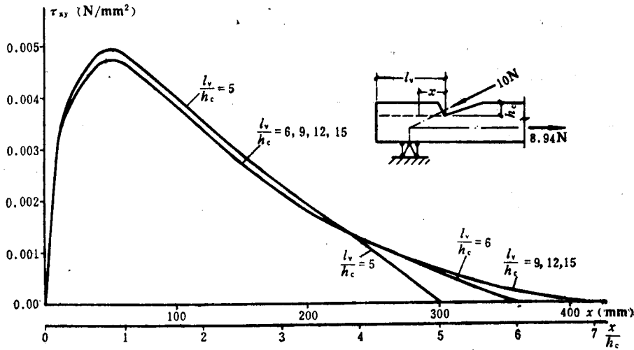
图 1-9 剪切应力 \tau_{xy} 沿剪面的分布状态
