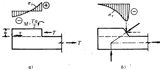
图 1-10 剪切面上横木纹方向的应力 \sigma ,
