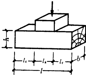
图 1-11 木材横纹承压
