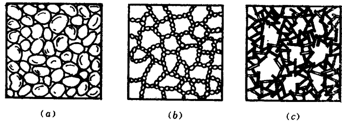
图 1-5 土的结构 (a) 单粒结构；(b) 蜂窝结构；(c) 绒絮结构
