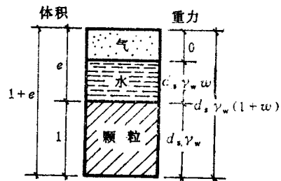
图 1-7 土的三相物理指标换算图
