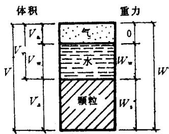
图 1-6 土的三相简图
