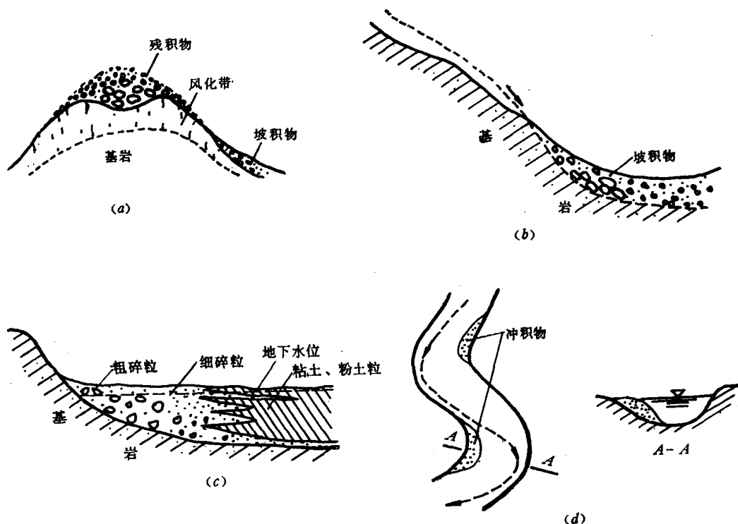
图 1-1 各种沉积土 (a) 残积土；(b) 坡积土；(c) 洪积土；(d) 冲积土
