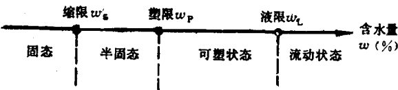
图 1-8 土的物理状态与含水量的关系
