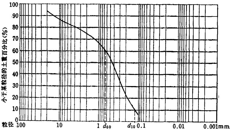
图 1-2 颗粒级配曲线示意图
