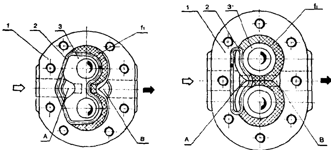
图 11 英国 Plessey 公司的间隙补偿结构
