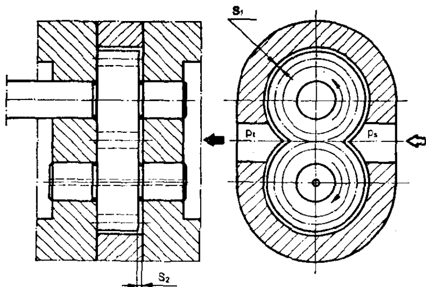
图 1 齿轮泵的结构
