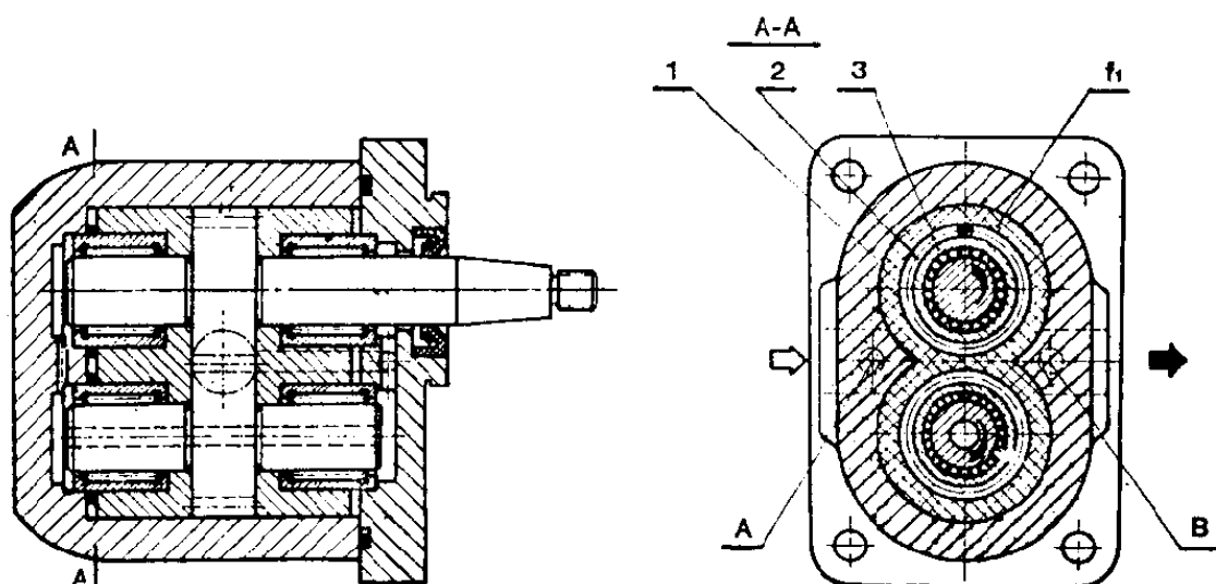
图7 轴向间隙补偿齿轮泵的结构
