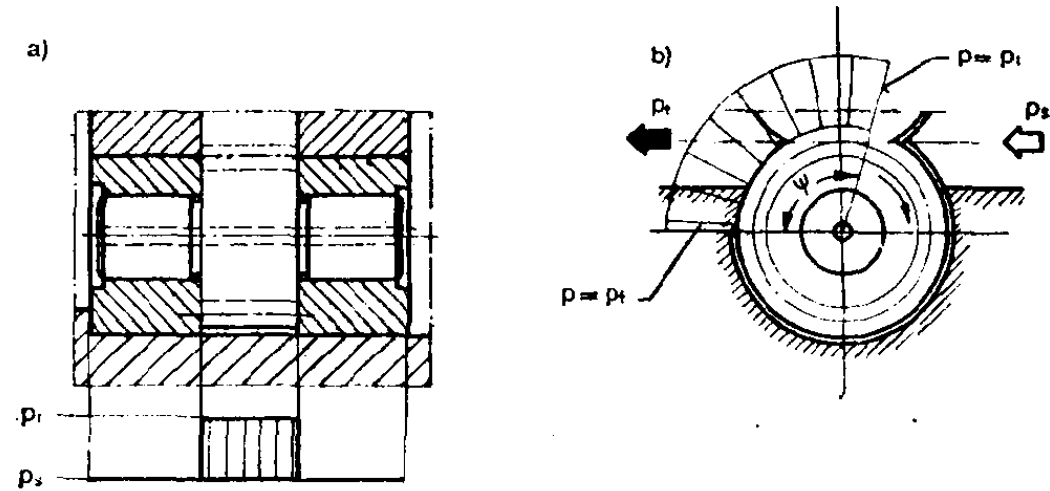
图 17 轴向间隙和径向间隙补偿齿轮泵的压力负荷图
