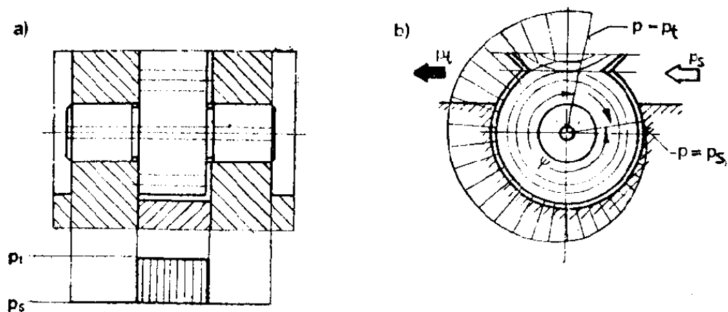
图6 轴向间隙补偿齿轮泵的压力负荷图
