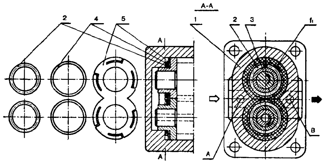
图 9 轴向间隙补偿齿轮泵
