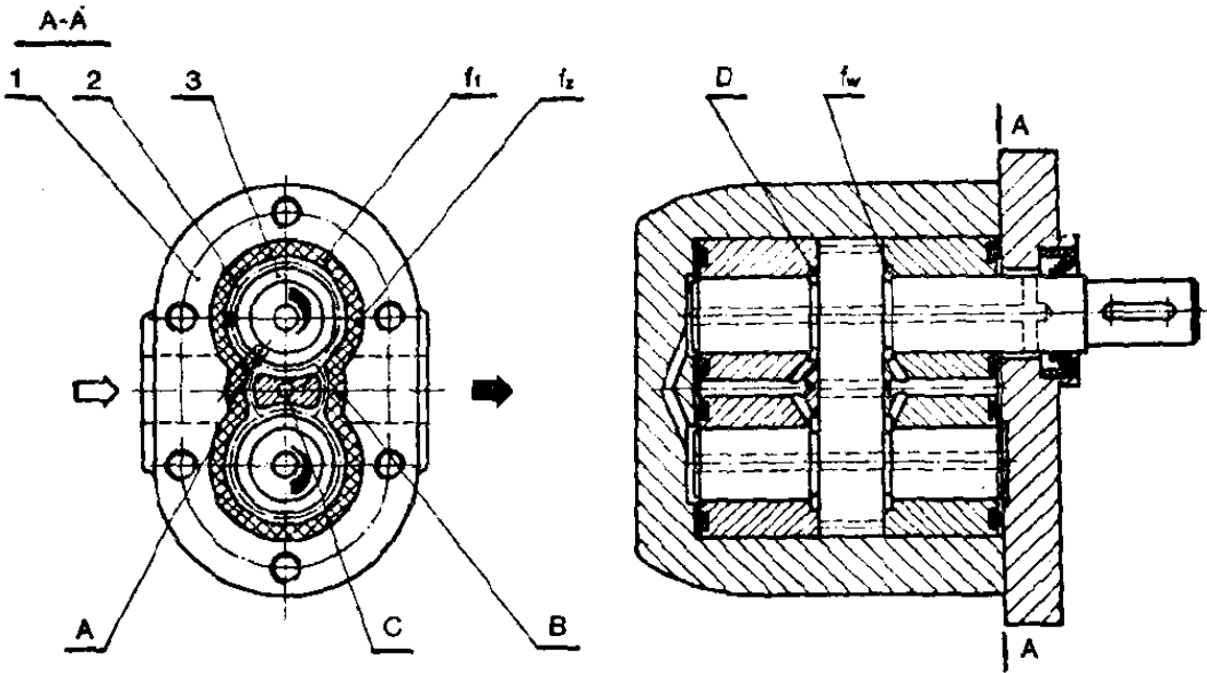
图 13 Bosch 公司的间隙补偿结构
