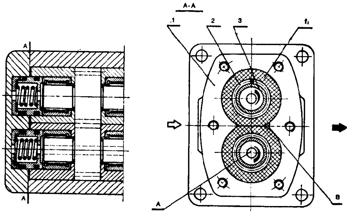
图 8 轴向间隙补偿齿轮泵
