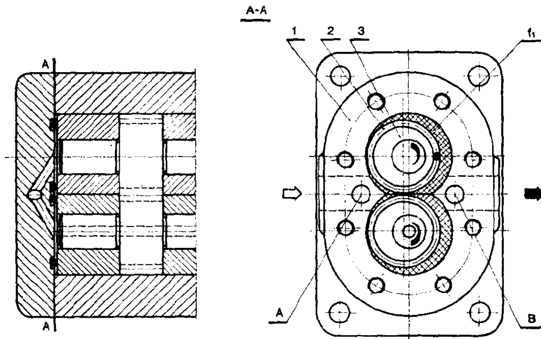
图 10 PZ 型齿轮泵间隙补偿原理
