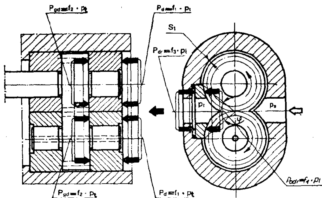
图 15 轴向间隙和径向间隙补偿齿轮泵的作用原理
