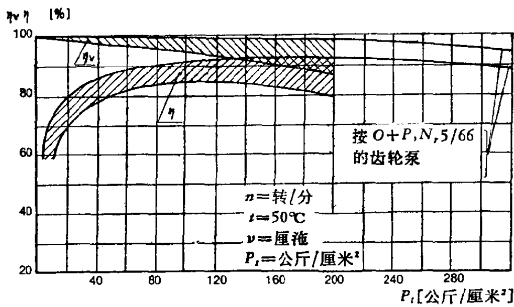
图 16 轴向间隙和径向间隙补偿齿轮泵的效率变化
