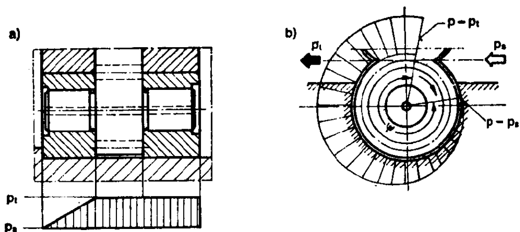
图3 固定间隙齿轮泵的压力负荷图
