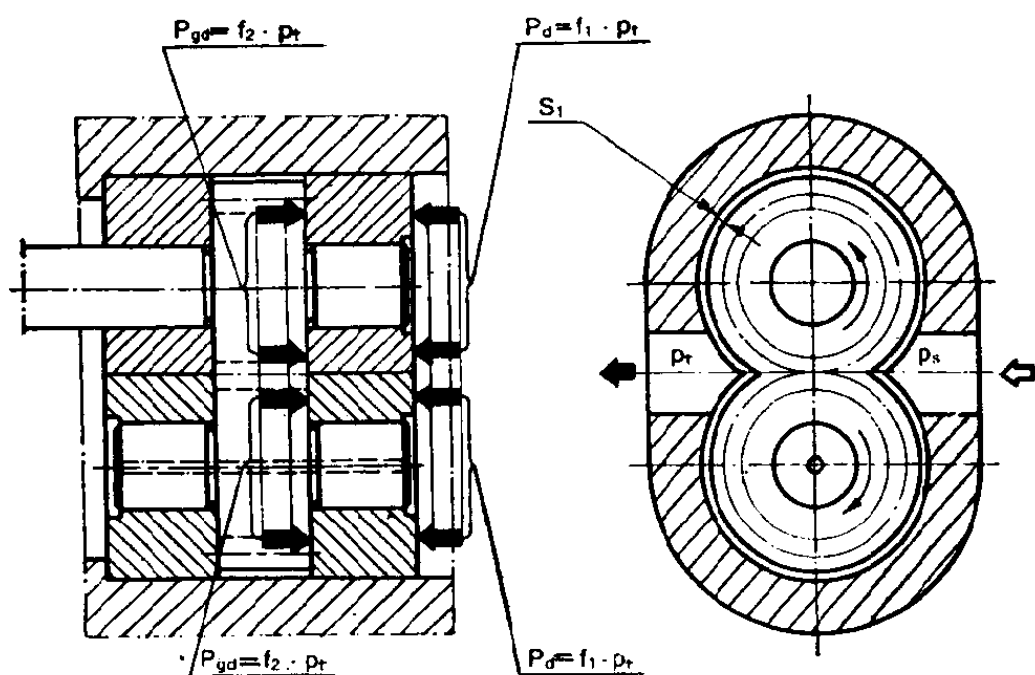
图4 轴向间隙补偿的作用原理
