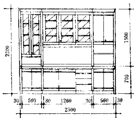
组合方案示例之三
