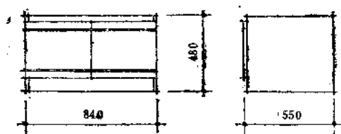
K型单元柜
