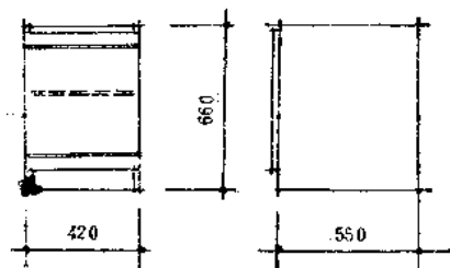
J型单元柜
