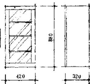
E1型单元柜
