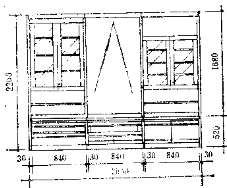
组合方案示例之八
