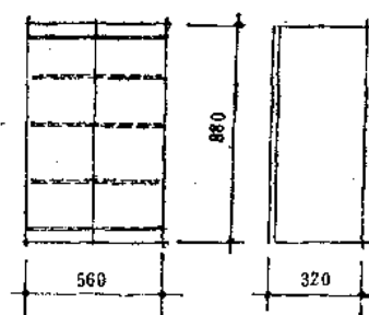
D型单元柜
