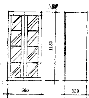
C型单元柜
