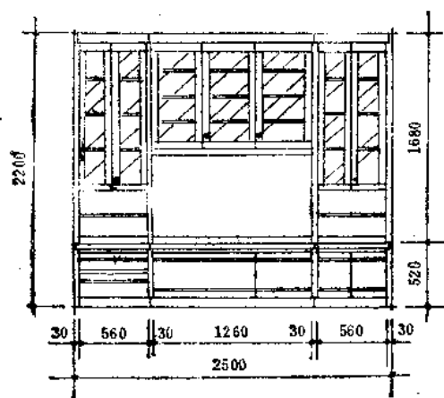
组合方案示例之五
