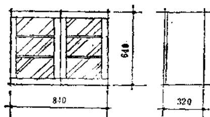
F型单元柜
