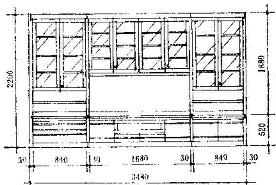
组合方案示例之一
