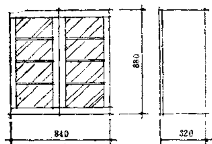
A型单元柜
