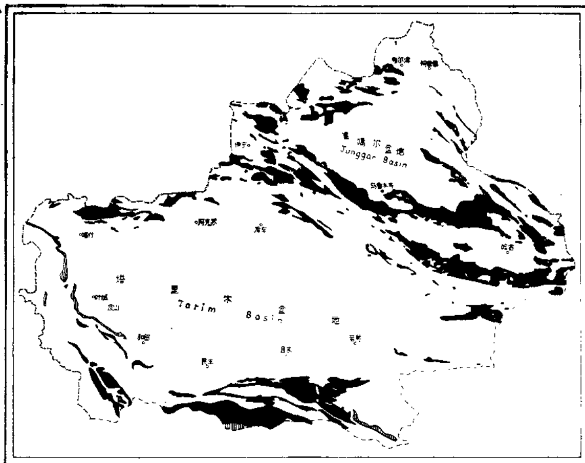
插图 1 新疆石炭系分布图
