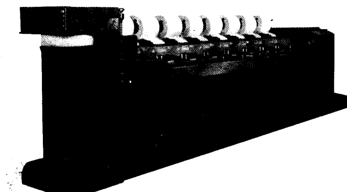
◀ 上海第一纺织机械厂生产的 FA251B 型棉精梳机是经改进后的一种新机型, 最高钳次数可达 230 钳次/分 纺织工业部技术装备司 供稿
