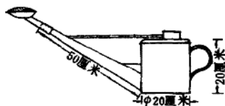
图 1 活头细眼喷壶示意图
