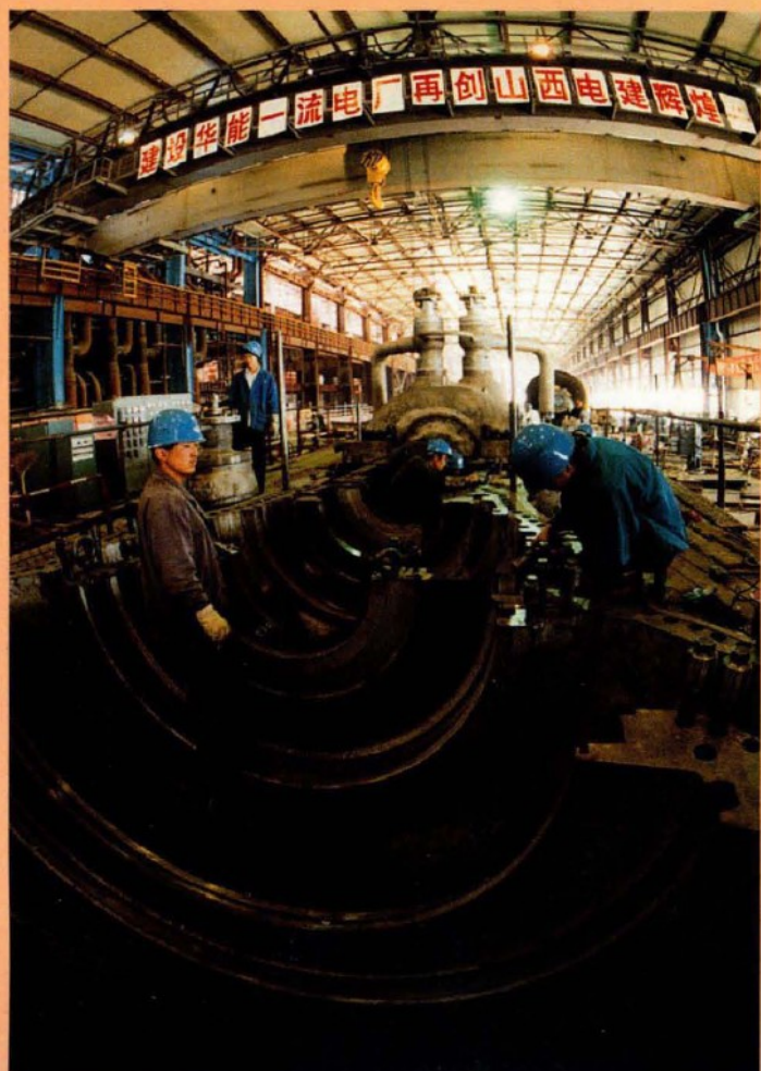
左：北京高碑店热 电厂机组安装
