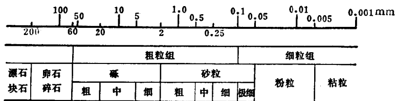
图 1-1 粒组划分图
