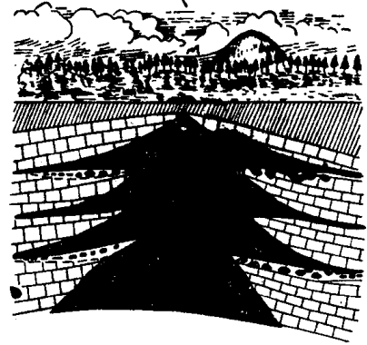
图 2—3 生物礁及其围岩的原始倾斜产状
