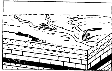
图 2—6 切割轻微时，地面只出露最新岩层
