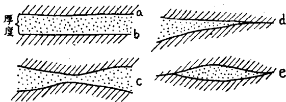
图 2-1 岩层的厚度和形态
