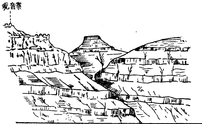
图 2—5 四川苍溪观音寨上侏罗统水平岩层素描图 (据李承三)
