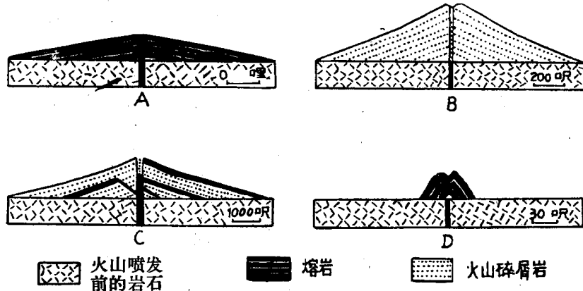
图 2—4 火山锥—火山碎屑岩及熔岩具原始倾斜
