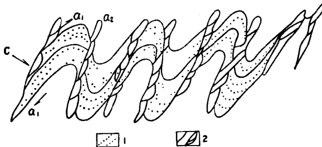
图 17 矿物沿滑移和转动面上的再分配
