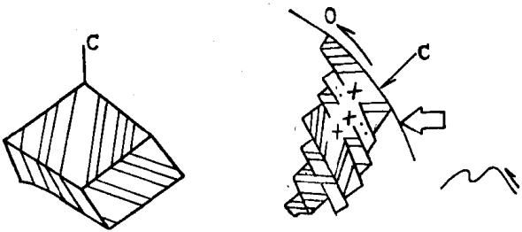
图 21 白云石沿 f ( 02\bar{2}1 ) 面塑性变形机制，转动后滑移
