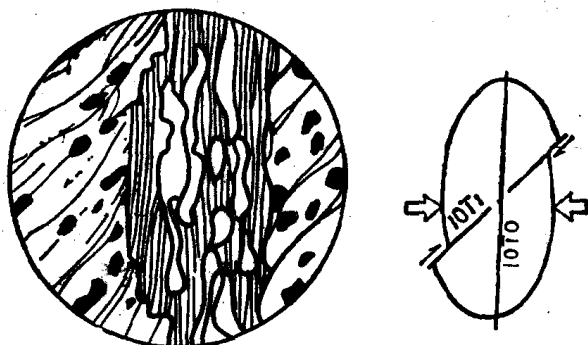
图 23 石英 (10\bar{1}0) 面与压性结构面平行定向
