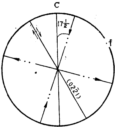
图 20 白云石的应变滑动
