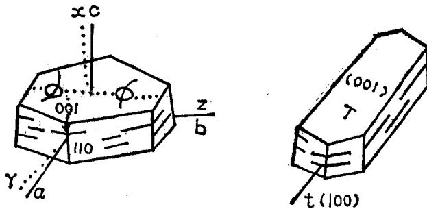
图 15 绢云母的光性方位和滑动系
