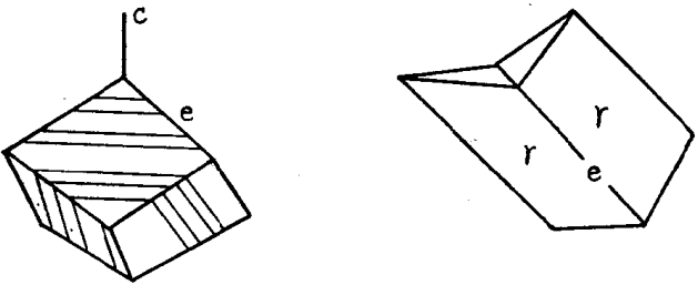
图 19 方解石沿 e ( 01\bar{1}2 ) 面的塑性变形机制
