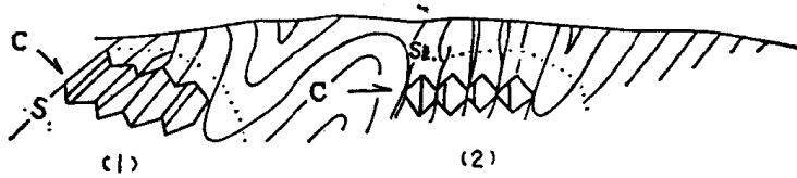
图 16 绢云母在不同边界条件下的运动
