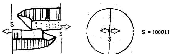
图 13 石英在张性结构面中的应力位
