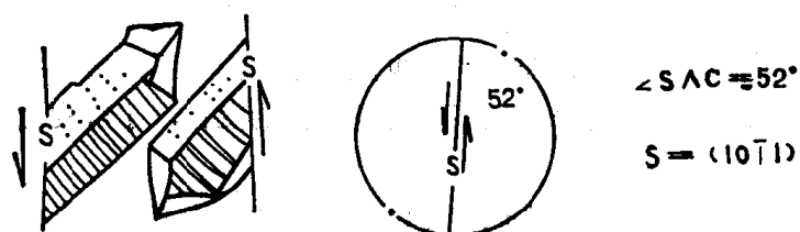
图 14 石英在扭性结构面中的应力位
