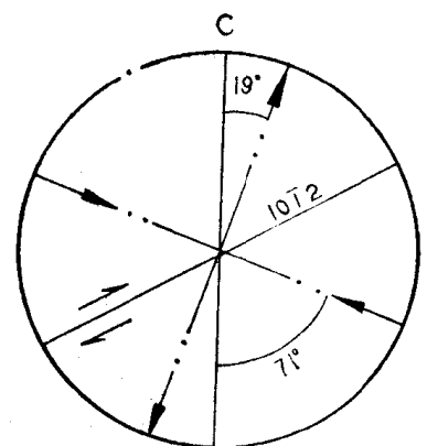
图 18 方解石的应变滑动
