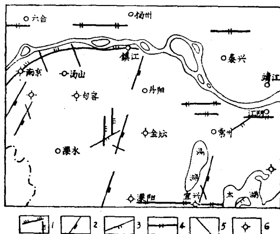
图1 苏南地区构造体系略图
