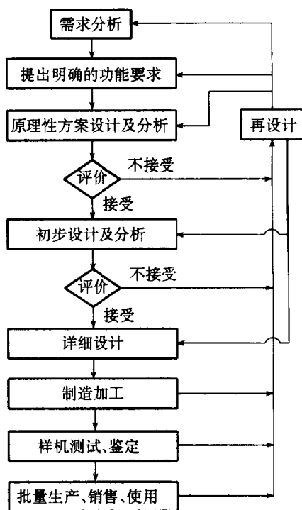
图 1-1 机械设计过程
