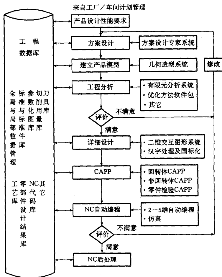
图 1-3 CAD/CAM 系统工作流程图
