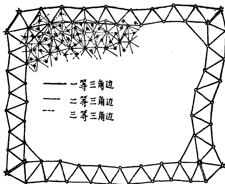
图1-11 国家一、二、三等网
