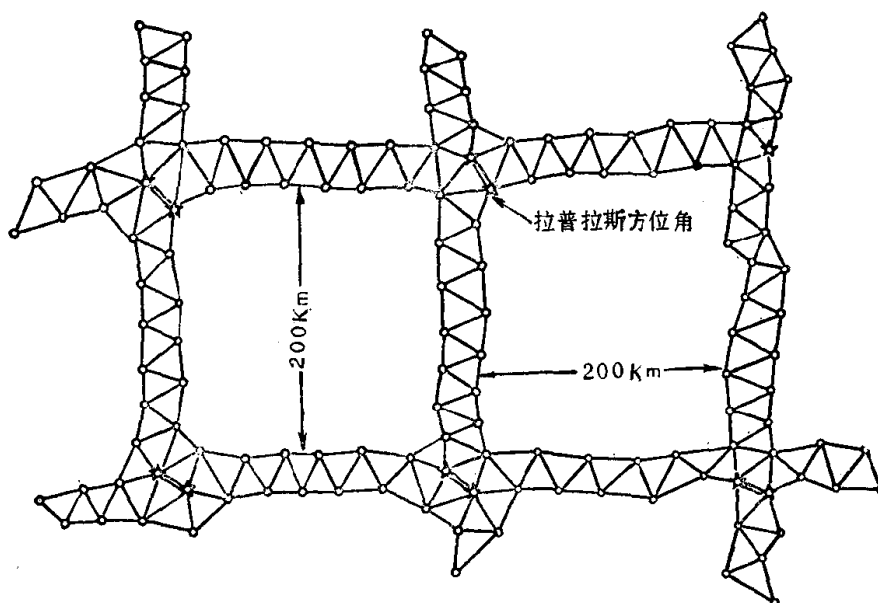
图1-10 国家一等三角锁
