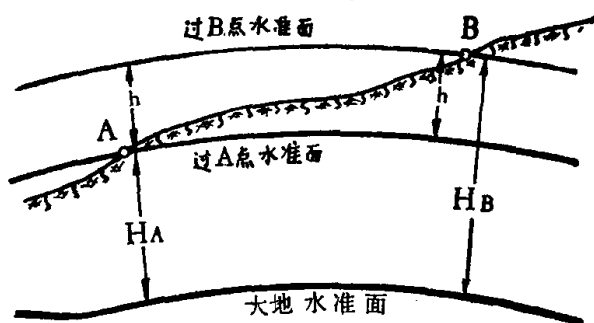
图1-7 高程和高差
