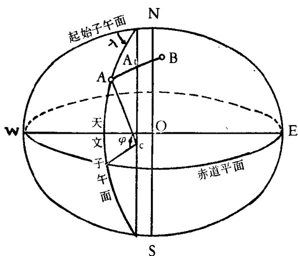
图1-5 地理坐标
