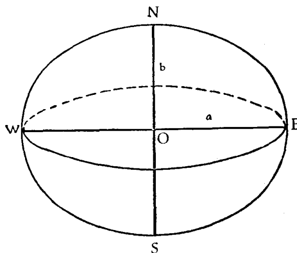
图1-4 参考椭圆体
