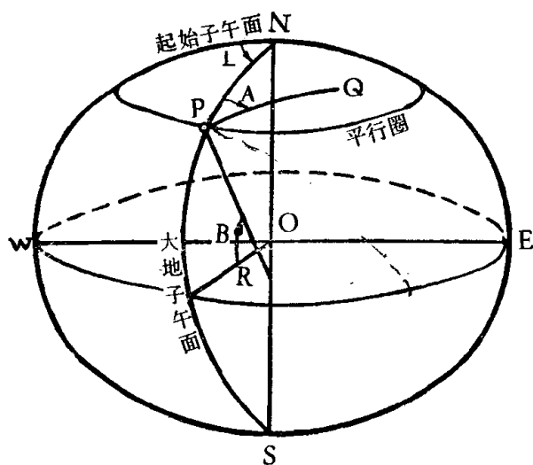
图1-6 大地坐标
