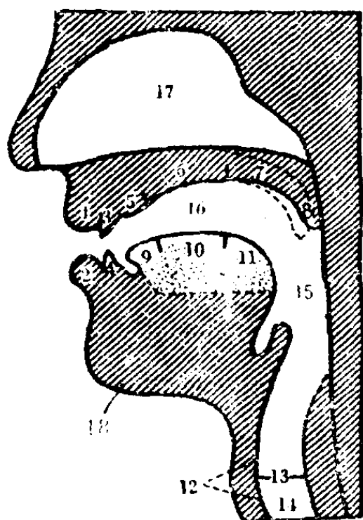
发音器官图
