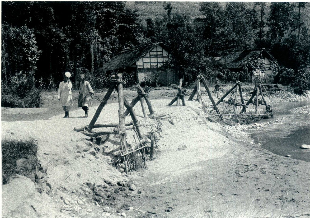
1917—1919 年，都江堰，拦水杓槎。
