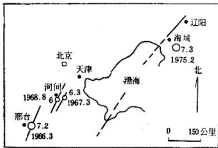
图 4 震中的迁移
