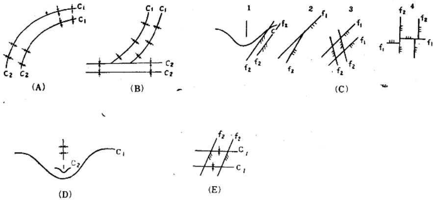
图 2 构造体系的复合
