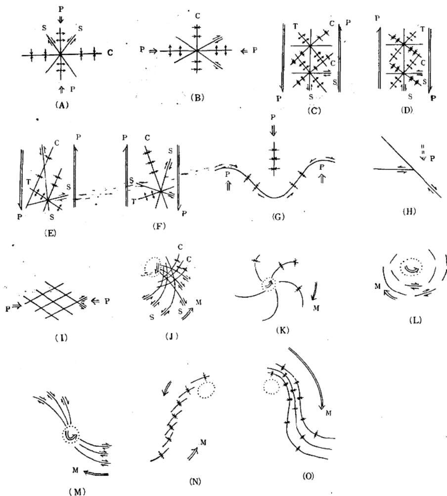
图 1 构造体系的型式
