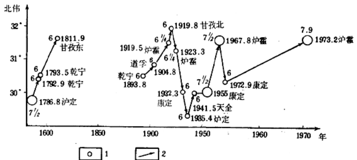
图 3 震中的迁移
