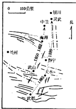
图 5 震中迁移
