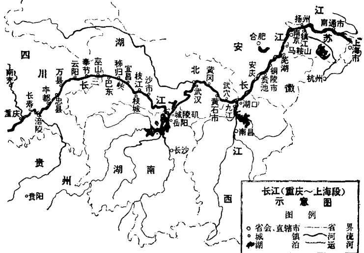
长江水系(重庆以下)图
