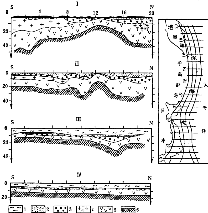
图5 从日本—千岛—堪察加岛弧向太平洋地壳结构变化图(据 Туезов, И. К. 1975)
