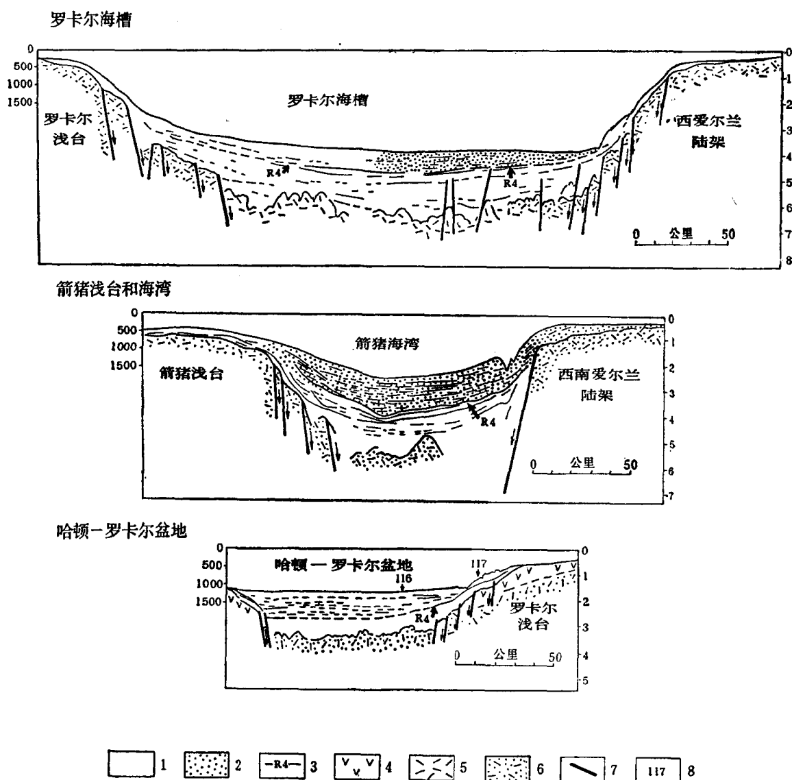
图7 罗卡尔海槽、箭猪海湾、哈顿-罗卡尔盆地地壳构造对比图(据 Raberts, D. G. 1974)
