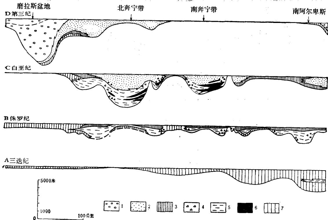
图6 中阿尔卑斯构造演化简图(据 Bernoulli, D. 等 1974)
