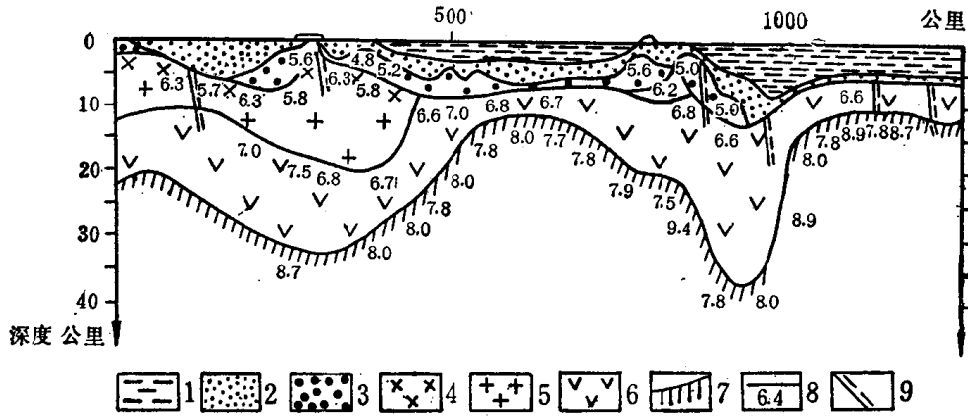
图4 横过萨哈林岛(库页岛)一千岛的地壳剖面(据 Туезов, И. К. 1975)
