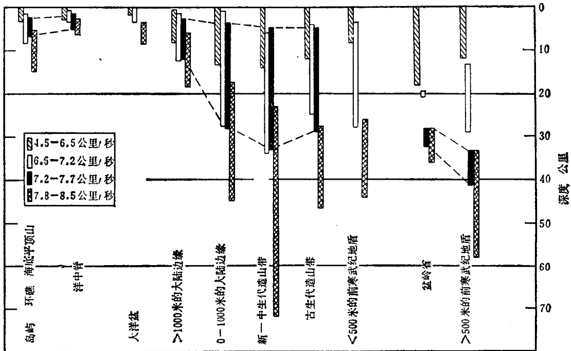
图 3 不同构造区的四种 P 波速度范围的深度(世界性数据的综合)(据 Drake, C. L. 等 1968) 四种速度范围相当于：4.5—6.5 公里/秒，上地壳；6.5—7.2 公里/秒，稳定的下地壳；7.2—7.7 公里/秒，构造活动区的不正常地壳或地幔；7.8—8.5 公里/秒，上地幔。
