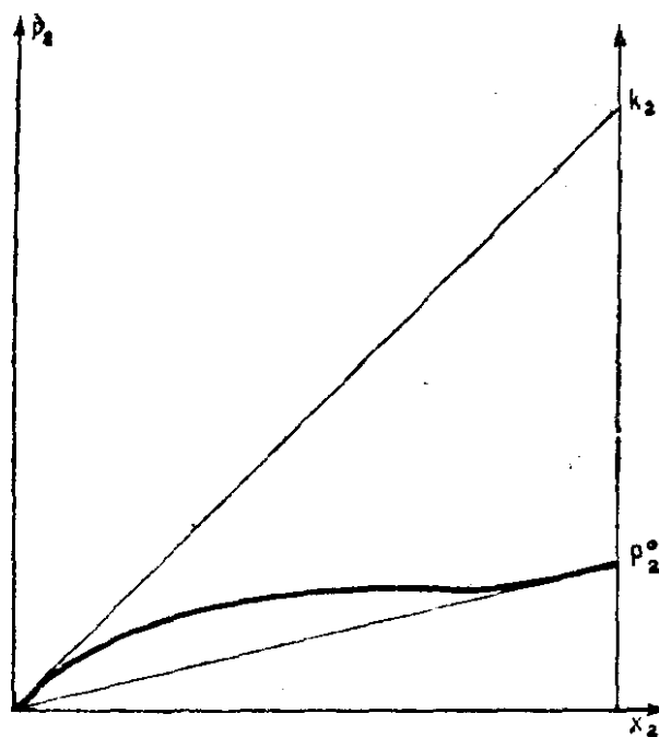
图 A.1.1 CS 2 在丙酮溶液的讨论图
