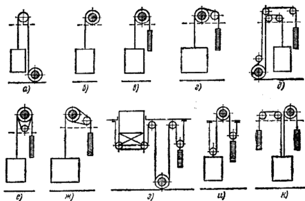
图3 电梯传动系统图
