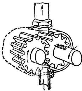
图 6 齿轮泵简图
