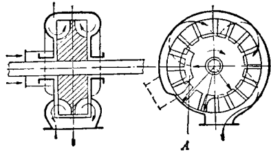
图 13 旋涡泵简图
