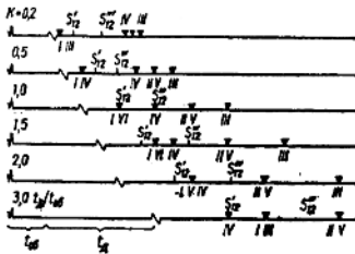
图11 超声波穿过传感器和岩样的时间（分别为 t_N 和 t_{0G} ）比值 ( K ) 不同时，纵波（I—VI）和横波信号入射和反射到压电接收器的时间图
