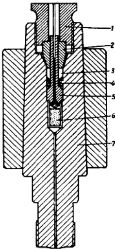
图 2 高压工作容器的一般外形
