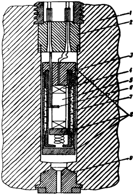
图4 高压容器的装配图
