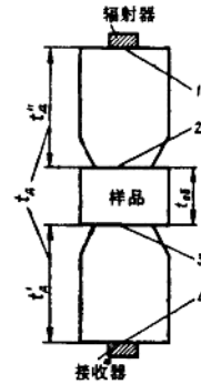
图10 传感器和岩样在高压室中的安装图 1—4 为超声波信号的反射面
