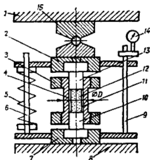
图6 按型槽法研究岩石的 ПИМ-7装置图
