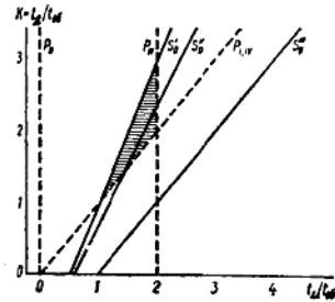
图12 t_N/t_{0G} 与 t_X/t_{0G} 的关系 S' 系 V_P/V_S = 1.5 时 S_0'' 系 V_P/V_S = 1.6 时， S_0''' 系 V_P/V_S = 2 时斜线区表示没有干扰的 可以测量 t_S 的范围
