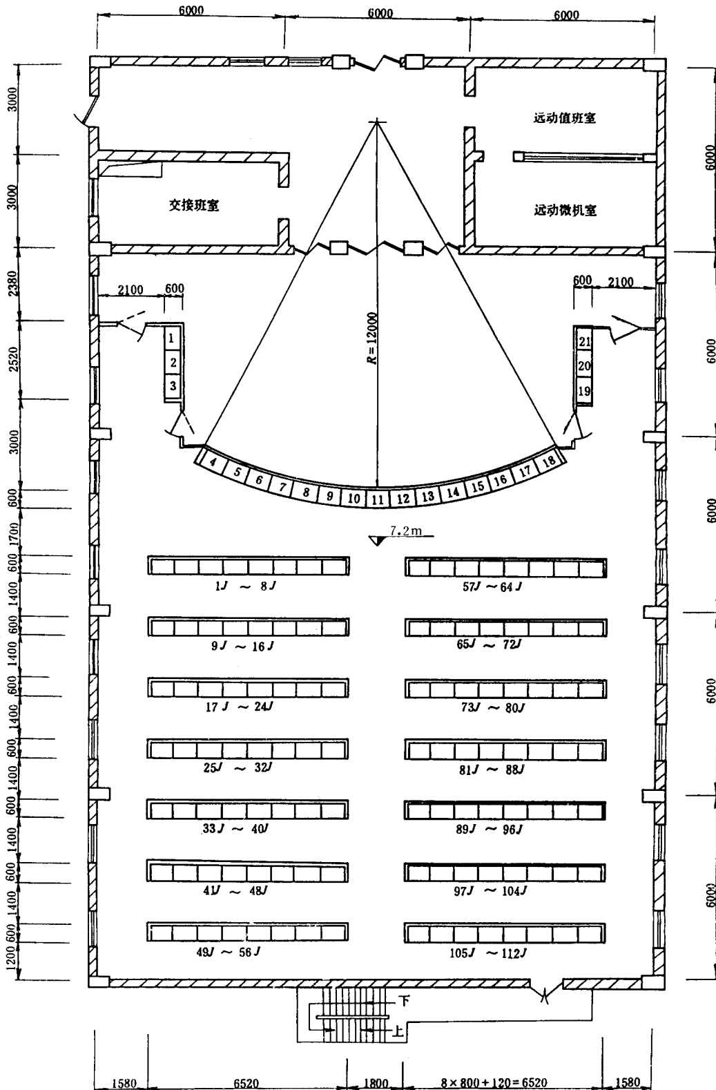
图 20-1 发电厂网控室布置方案一
