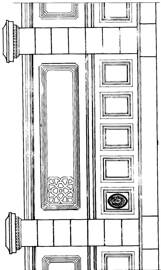
立面图
