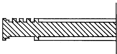
剖面图
