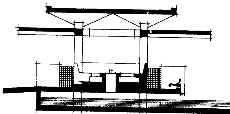
图1 剖面
