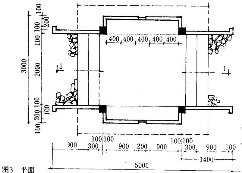
图3 平面
