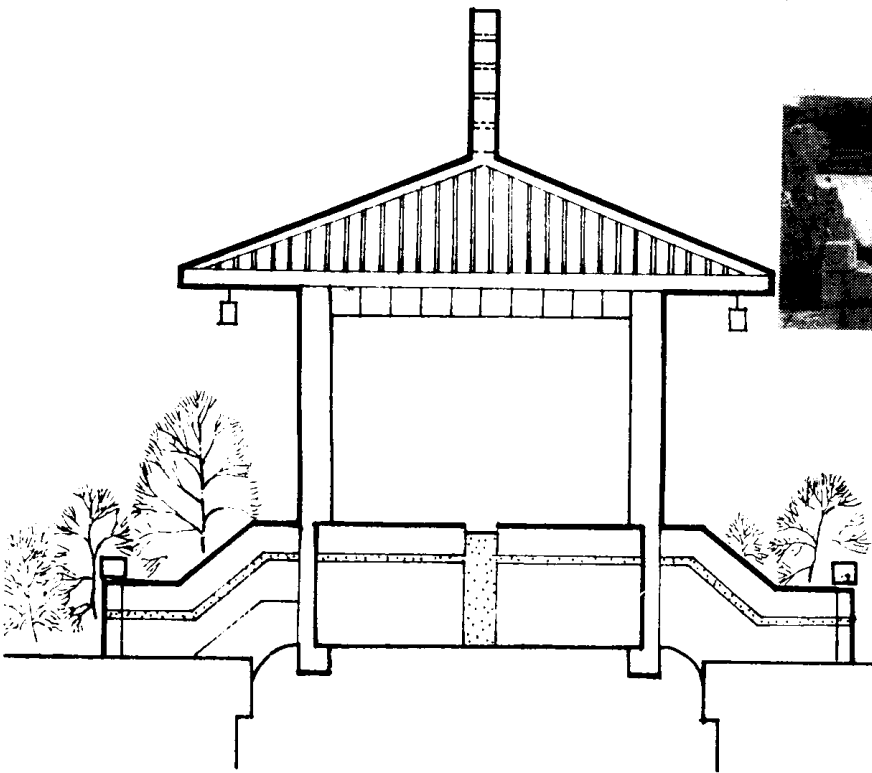
图2 侧立面
