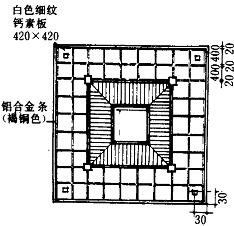
图7 天棚平面
