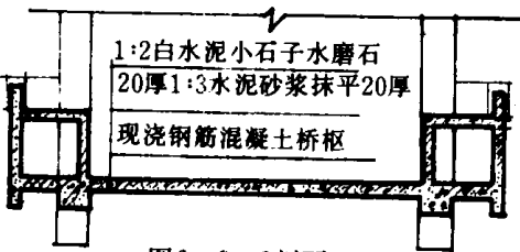
图6 2—2剖面
