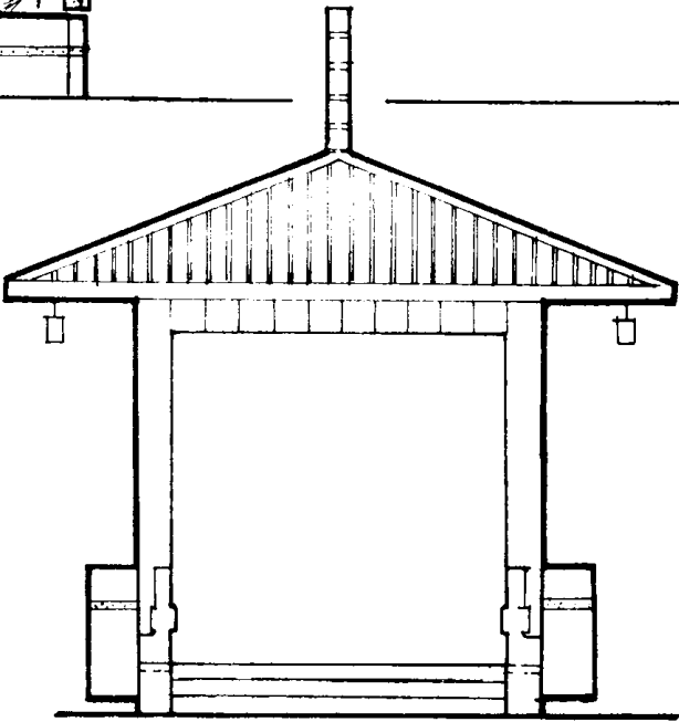
图4 正立面
