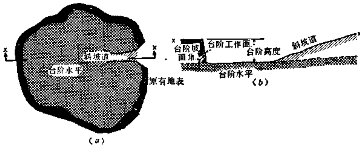
图 9-2 单台阶开采的露天矿
