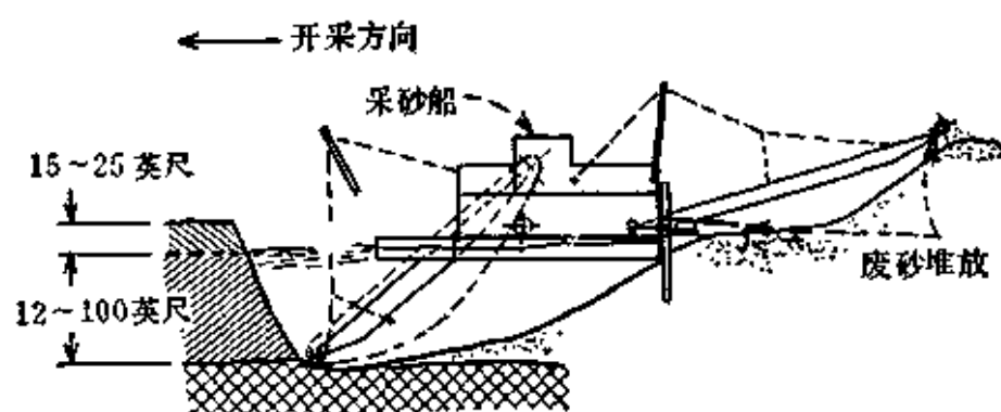
图 9-1 采砂船开采
