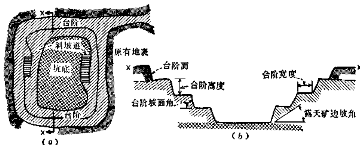
图 9-3 多台阶开采的露天矿
