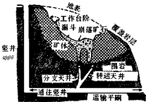
图 9-6 漏斗式开采 (1)
