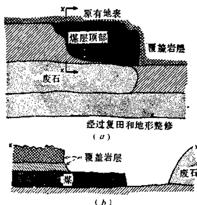
图 9-4 剥离露天矿
