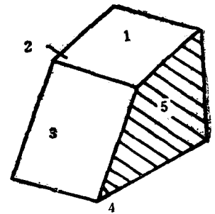
图2—1 斜坡的组成 1—坡顶面；2—坡肩； 3—坡面；4—坡角； 5—坡体
