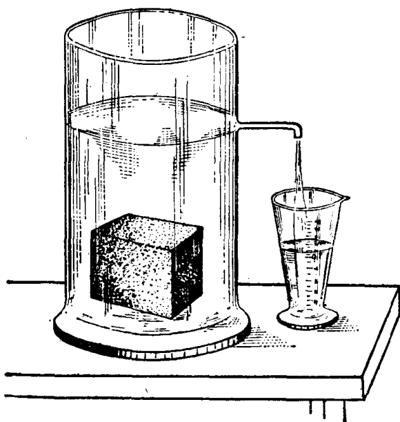
图 1·10 量度较大固体的体积
