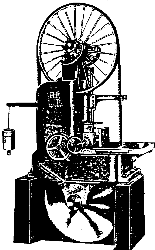
MJ 3310 A平台式木工带锯机床
