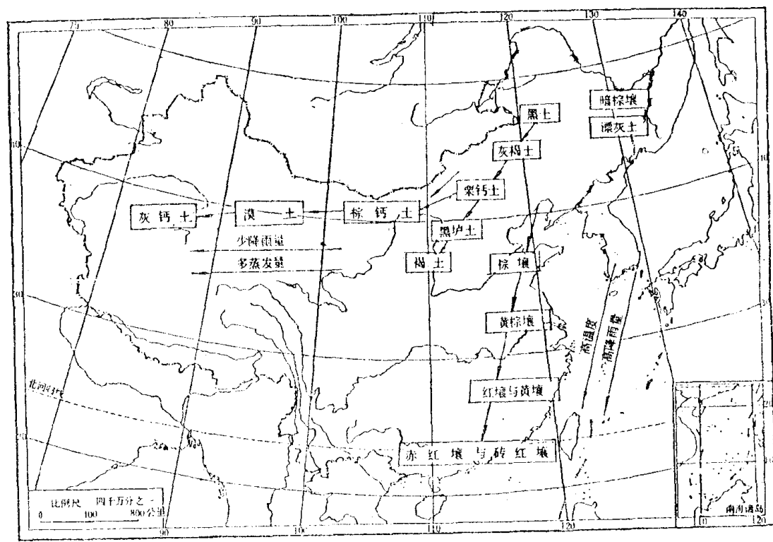
图 1-1 我国土壤水平地带分布示意图
