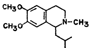
(14) \lambda \sim 285\text{nm}
