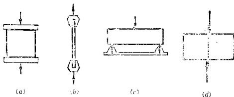
图 1-1 材料强度试验示意 (a)压力；(b)拉力；(c)弯曲；(d)剪切
