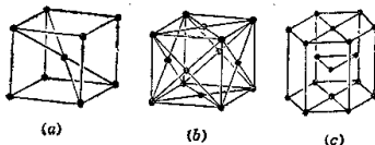
图 1-7 结晶格子
