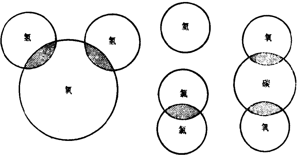
图 1-1 分子由原子组成。一个水分子由两个氢原子和一个氧原子组成。一个氮分子由一个原子组成。一个氮分子由两个原子组成。一个二氧化碳分子由三个原子组成。
