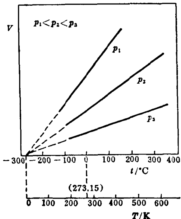
图1-3 理想气体的 V-T 图
