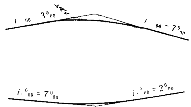
图 1—1—8 竖曲线示意图
