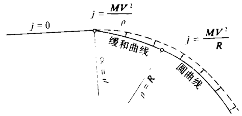
图 1—1—4 缓和曲线示意图
