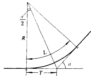
图 1-1-3 圆曲线要素图
