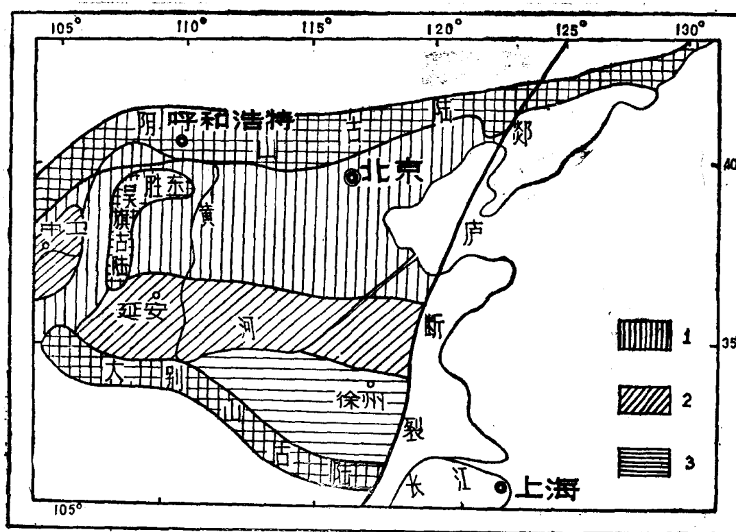
图2 华北陆台石炭一二叠纪煤系地层分布图
