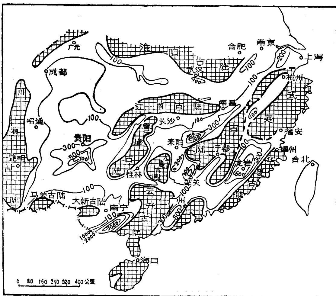
图1 华南晚二叠世龙潭组等厚图(据韩德馨等)
