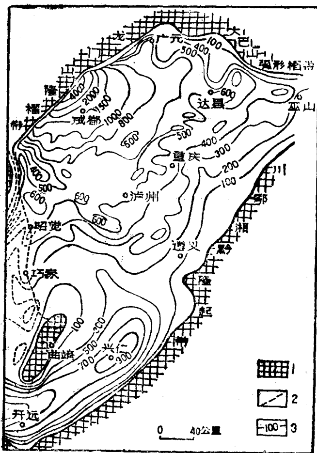
图3 华南西部晚三叠世含煤沉积等厚图(据韩德馨等) 1—古隆起带; 2—川滇隆起带界线; 3—等厚线
