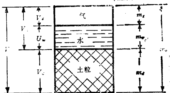
图 2-3 土的三相简图
