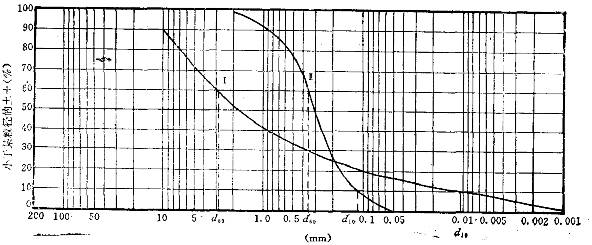
图 2-1 粒径极配曲线
