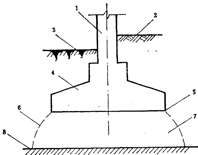
图 1-2 地基基础示意图
