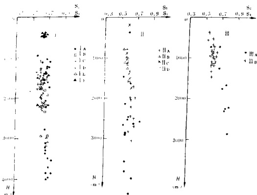
图 1-10 I A—III B——地应力测点位置
