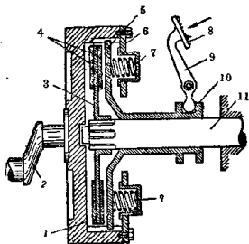
图 1-7 常压式离合器简图
