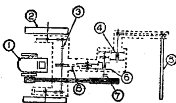
图 1-3 耕耘机传动系
