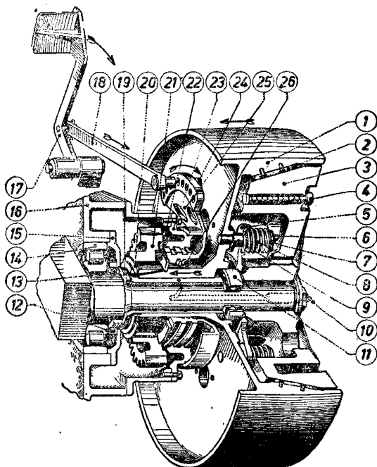
图 1-11 SL50/55 型拖拉机的离合器
