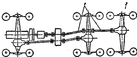
图 1-6 解放牌 CA-30 (ЗИЛ-157) 汽车传动系
