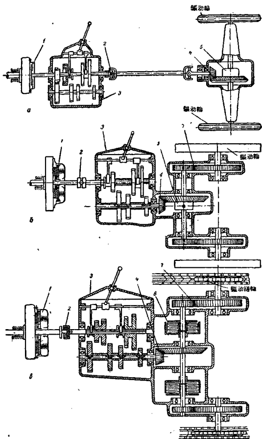
图 1-1 拖拉机汽车传动机构简图
