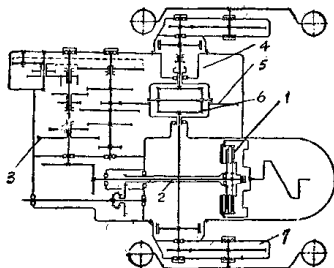
图 1-2 自动底盘传动系
