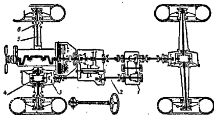
图 1-5 格斯-63 汽车的传动系
