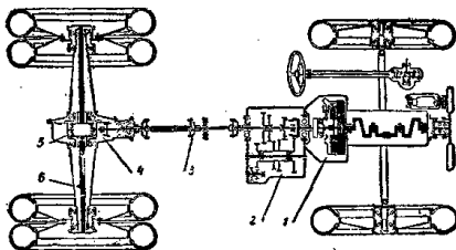
图 1-4 跃进牌汽车的传动系
