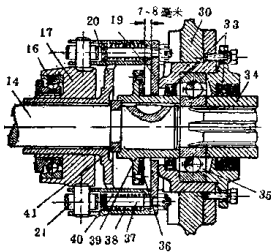
图 1-9 东方红-54 拖拉机离合器的小制动器装置
