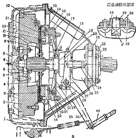
图 1-8 东方红-54 拖拉机的离合器
