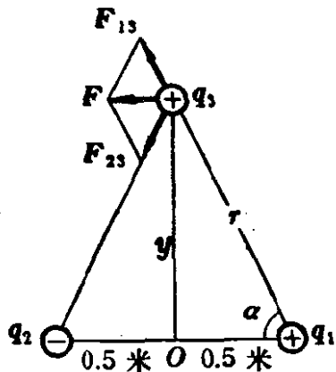
图 4-1-3 静电力迭加举例
