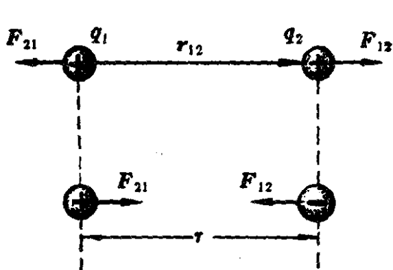
图 4-1-1 两点电荷的相互作用
