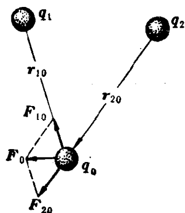
图 4-1-2 静电力的可迭加性
