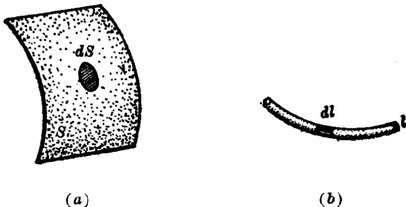
图 4-1-5 电荷面密度(a)和电荷线密度(b)
