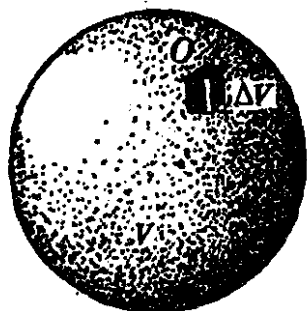
图 4-1-4 体电荷密度
