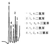
图1 氯苯类化合物的气相色谱图
