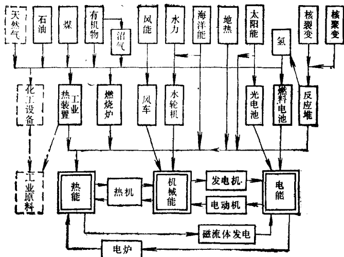
图1-1 能源的转化和应用
