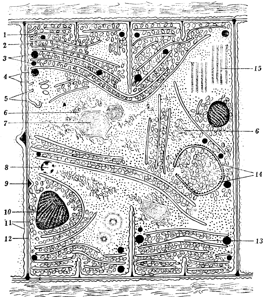
图 1-1 电子显微镜下蓝藻细胞的构造
