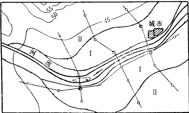
图 1-2 河流冲积平原勘探线布置示意图
