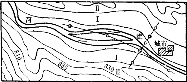
图 1-1 山间河谷勘探线布置示意图
