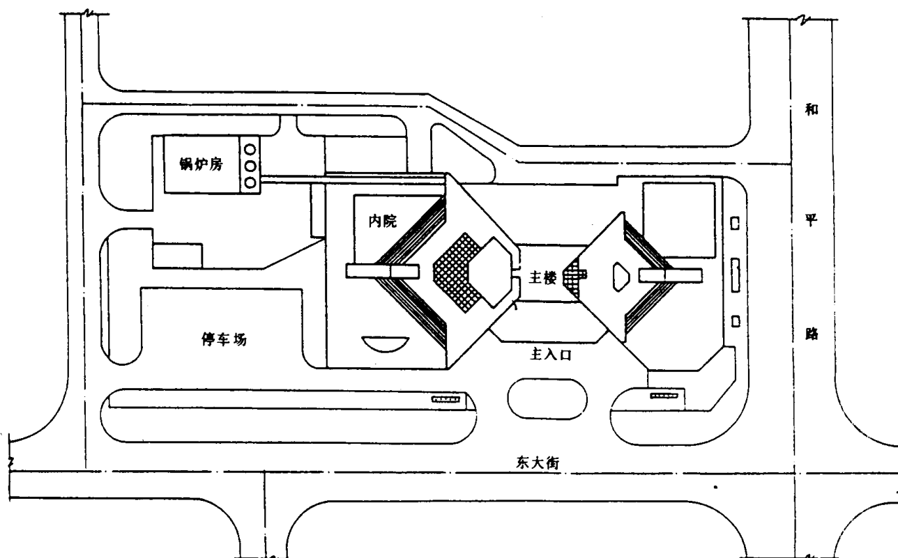
总平面
