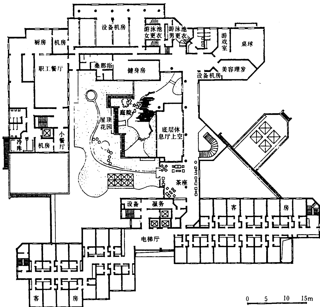
二層平面
