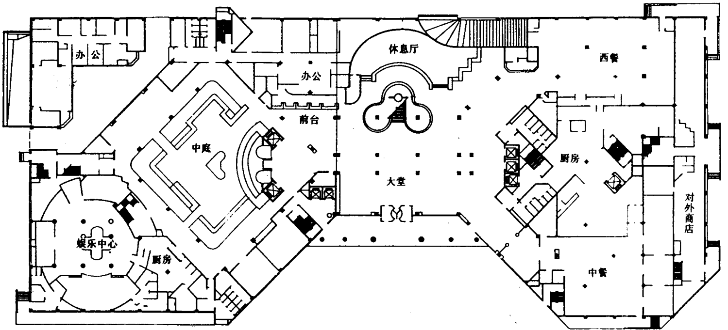
首层平面
