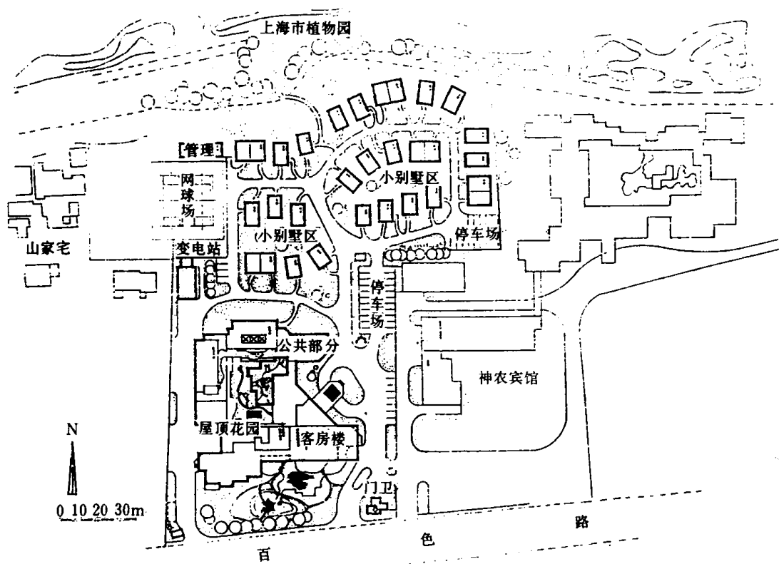
总平面
