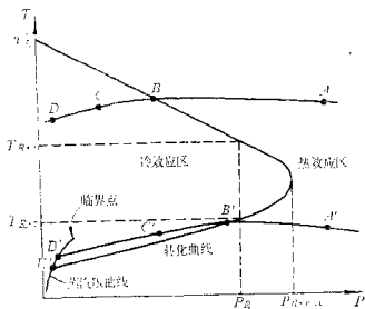
图 3-6 T-P 图示节流过程
