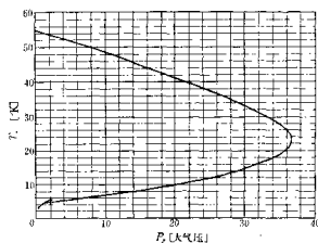
图 3-3 氩的转化曲线 (22)
