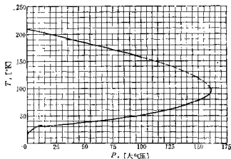
图 3-5 仲氢(p-H 2 )的转化曲线 (24)
