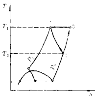
图 3-1 节流过程在 T-S 图上的表示
