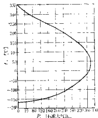
图 3-2 氮的转化曲线 (21)
