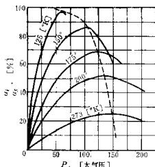
图 3-8 空气的 \frac{\alpha_i}{\alpha_i} 与 T 、 P 的关系 (21)
