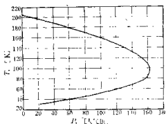
图 3-4 标准氢的转化曲线 (23)
