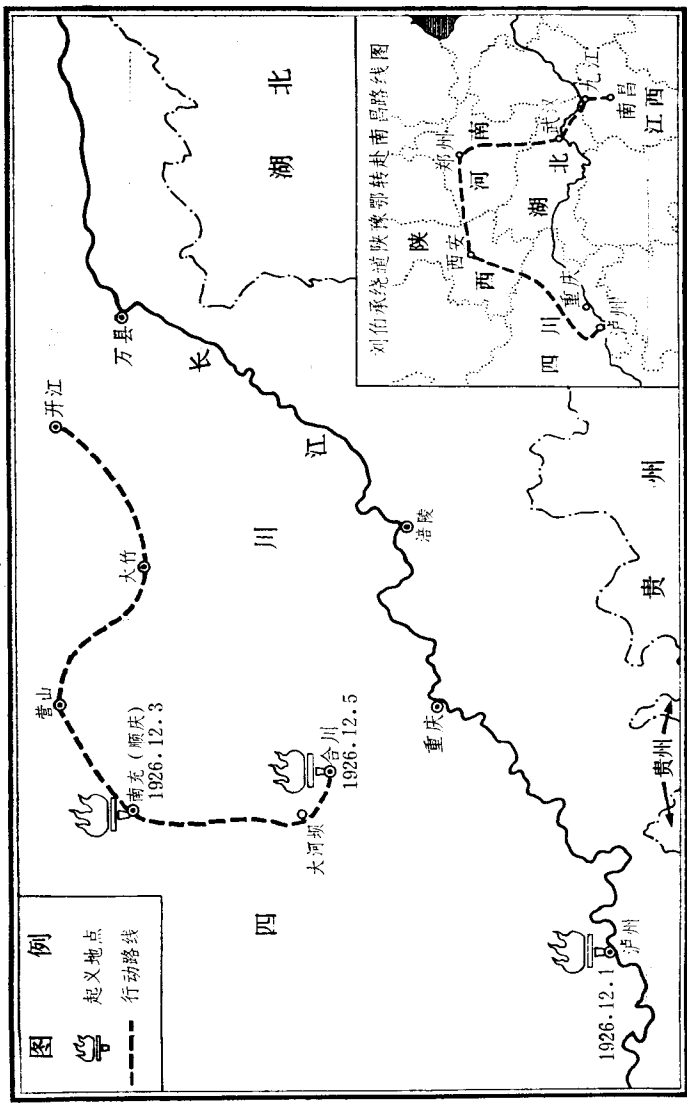
泸州顺庆起义形势图
