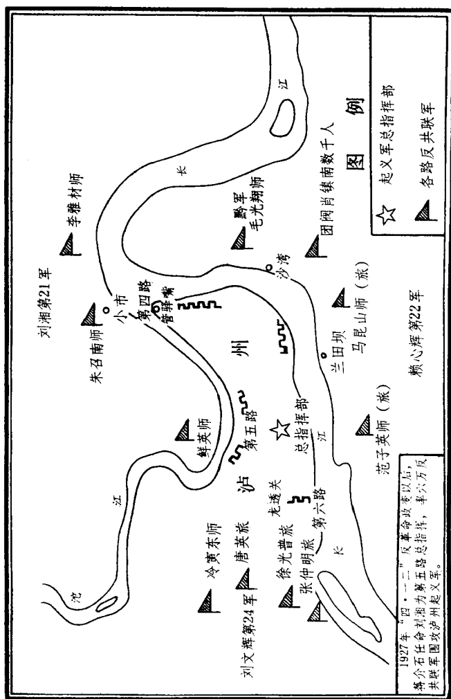
泸州守城战敌我态势图
